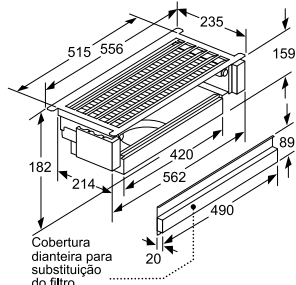
Instalação do exaustor integrável com módulo Clean Air
