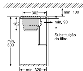
Instalação do exaustor integrável com módulo Clean Air
