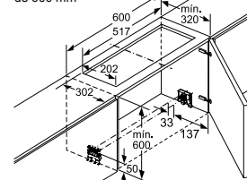
Instalação do exaustor em móvel de 600 mm
