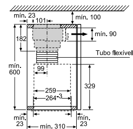
Instalação da caixa do exaustor telescópico com módulo Clean Air
