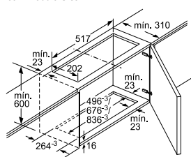
Instalação da caixa do exaustor integrável com módulo Clean Air
